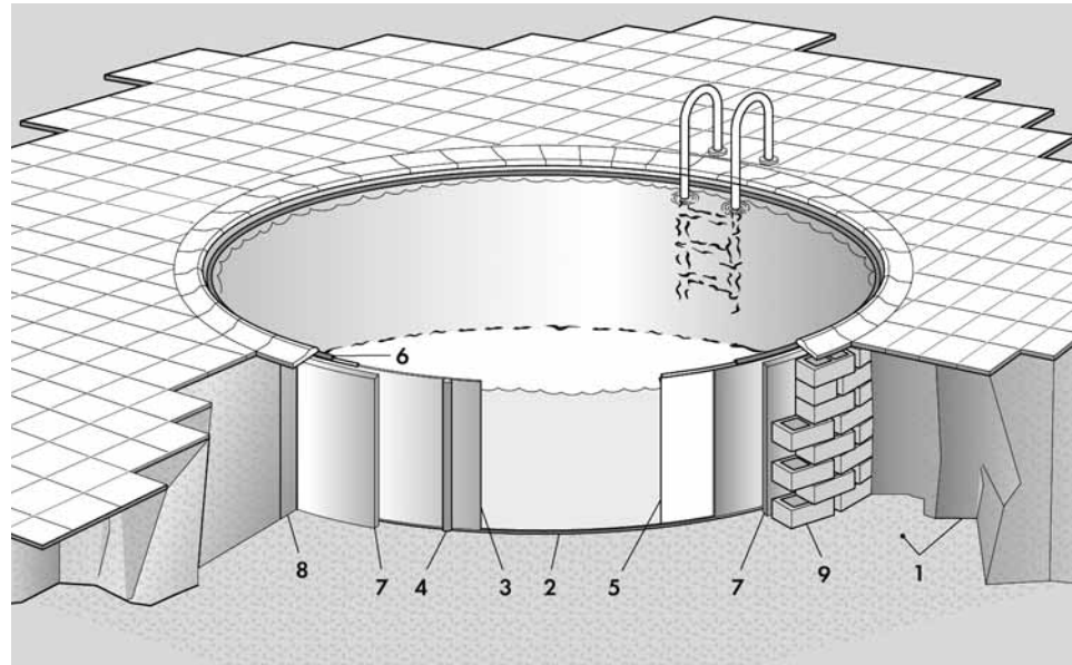
Tiefbecken mit Hinterfüllung aus Magerbeton (links) oder alternativ mit Mauerwerk (rechts)
